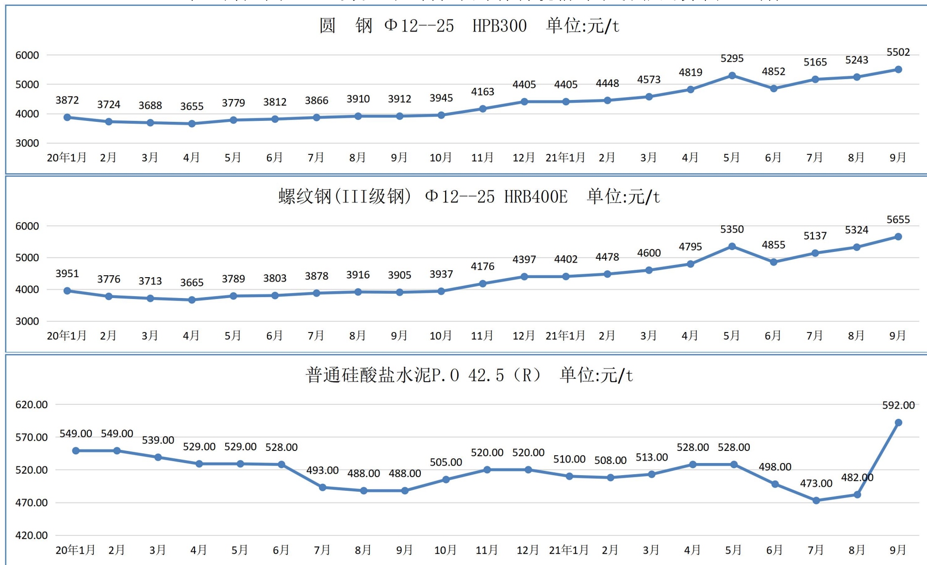
2021 年 9 月广州地区建设工程部分常用材料税前综合价格走势（试行）
