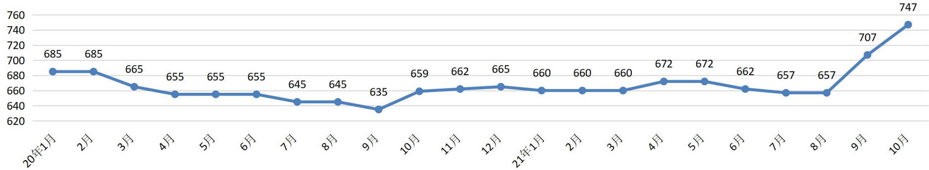
湿拌抹灰砂浆 M20 单位:元/m 3
