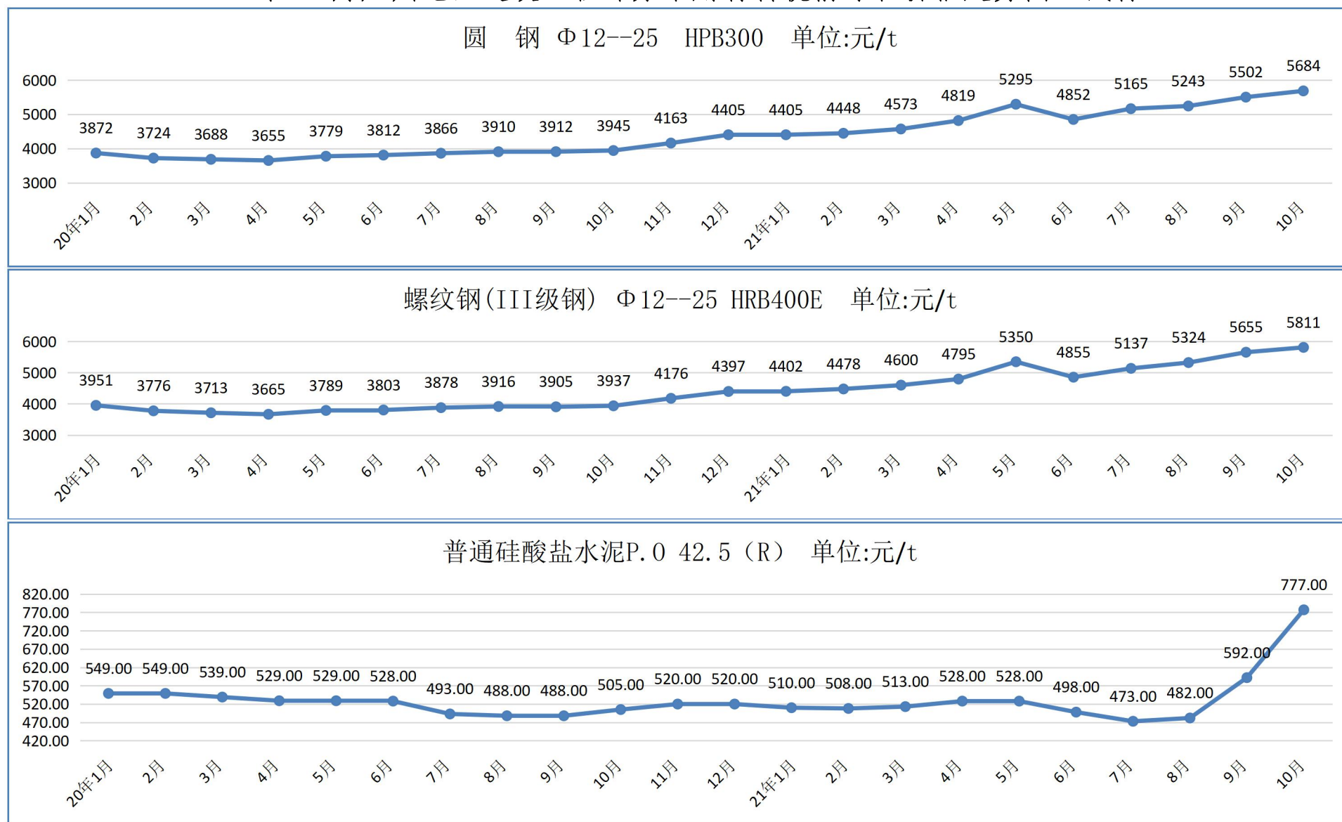
2021 年 10 月广州地区建设工程部分常用材料税前综合价格走势（试行）
