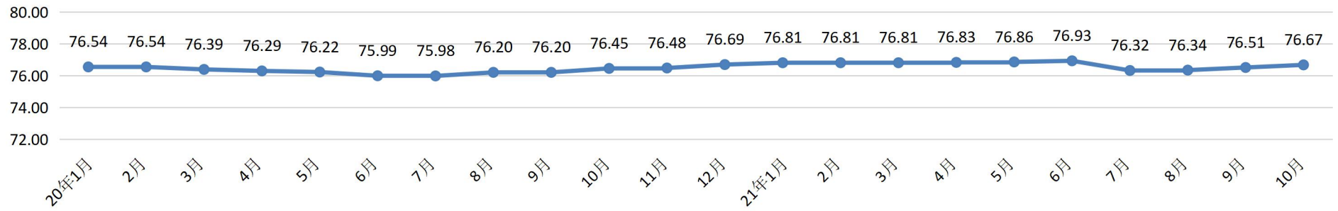
普通泵送混凝土 C30 单位:元/m 3
