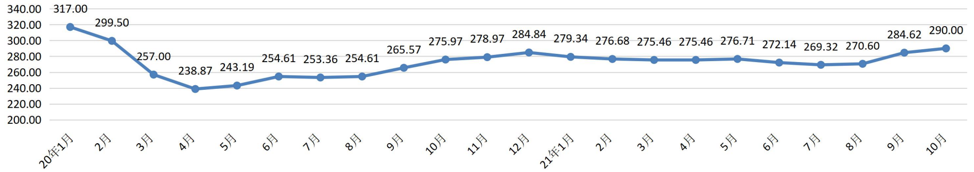
机 制 砂 单位:元/ m 3
