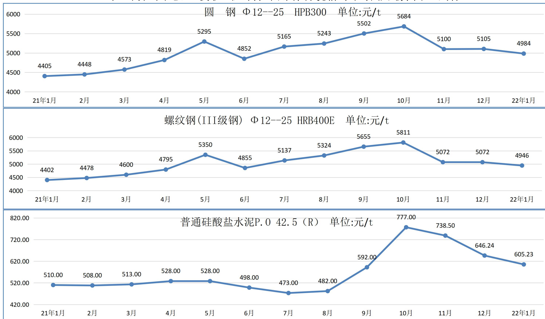
2022 年 1 月广州地区建设工程部分常用材料税前综合价格走势（试行）
