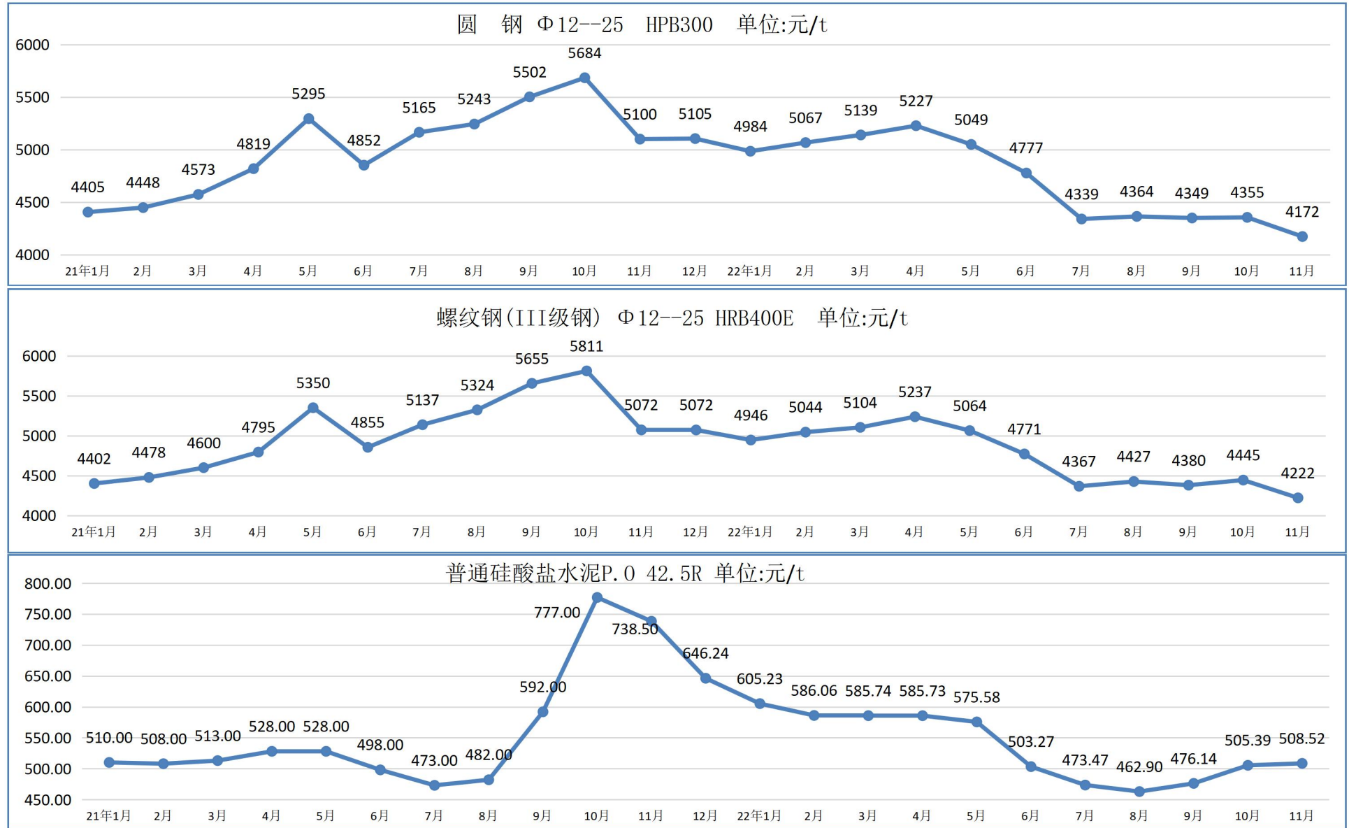
2022 年 11 月广州地区建设工程部分常用材料税前综合价格走势图（试行）
