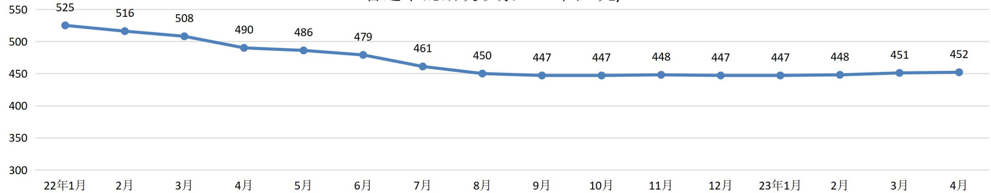
湿拌砌筑砂浆 M5 单位:元/m 3
