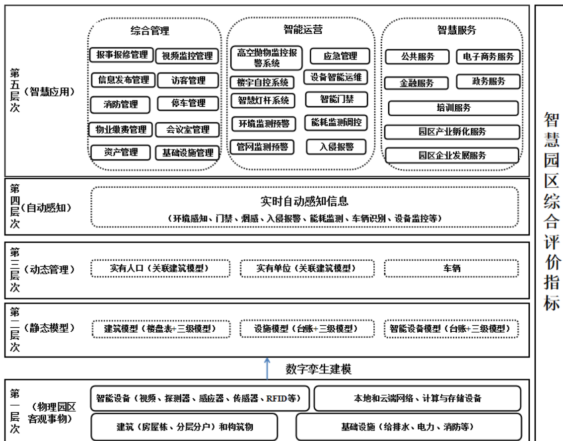
图 3.1.1 基于 CIM 的智慧园区总体框架
