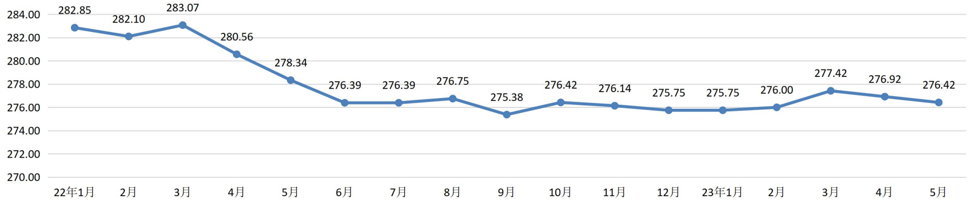
中 砂 细度模数 3.0—2.3 单位:元/m 3
