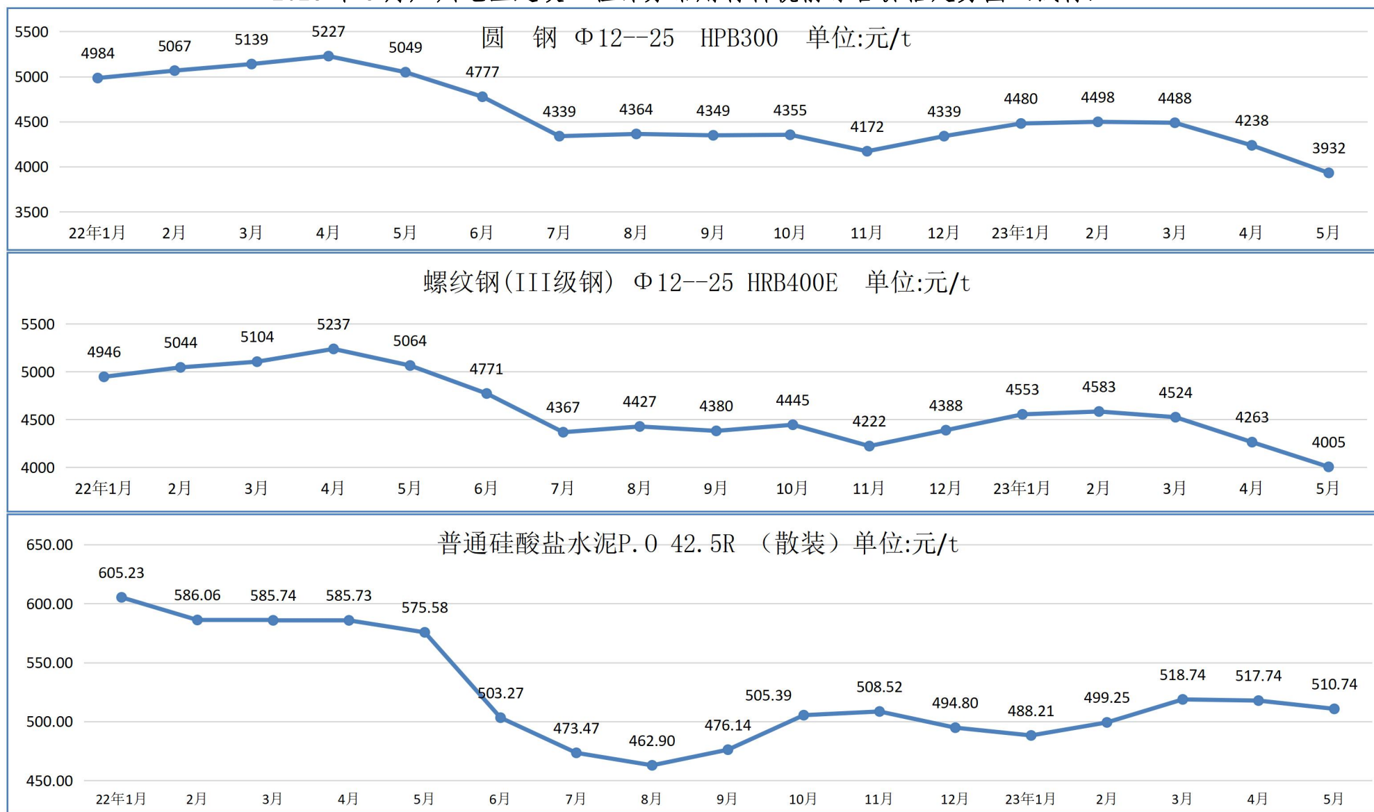
2023 年 5 月广州地区建设工程部分常用材料税前综合价格走势图（试行）
