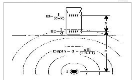
图 7 直读法
