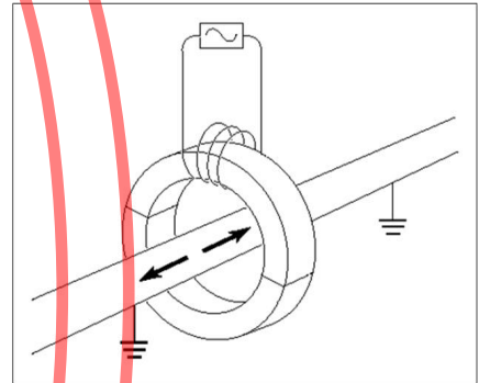
图3 夹钳法
