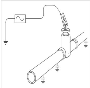
图1 直连法
